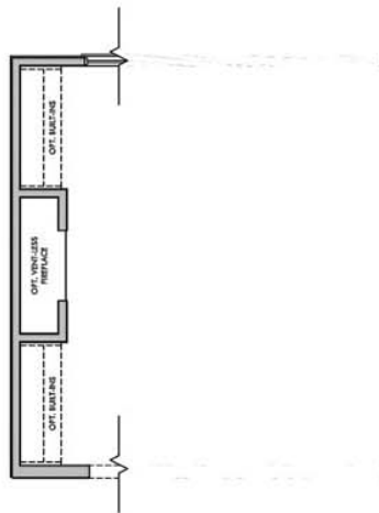
FIREPLACE OPTION SCALE: 1/4" = 1'-0"
